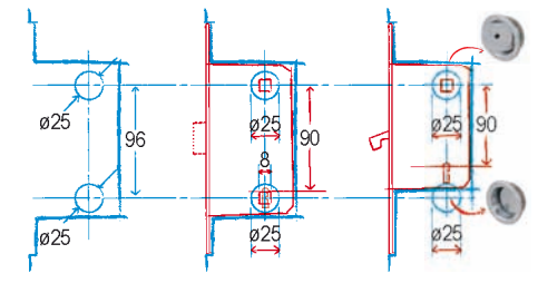
Freziranje krila Sash drilling Mediana i XT Mediana and XT Scivola T Mediana čelo Scivola T Mediana forend
