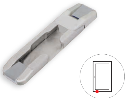
Prihvatnik otklopa sa podiznim klinom Tilt striker with lifting wedge
