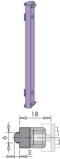
Distanzstück A0085
