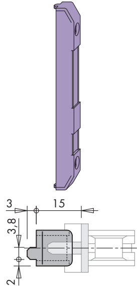
Distanzstück A0085
