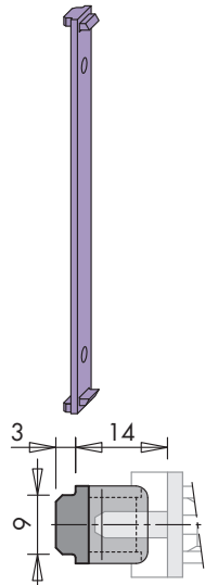
Distanzstück A0105
