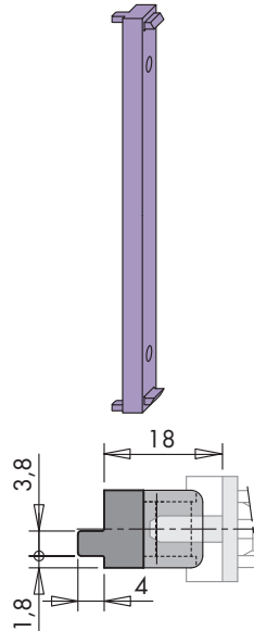
Distanzstück A0157
