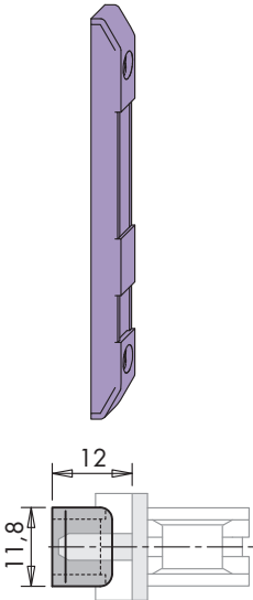
Standard Schließblech
