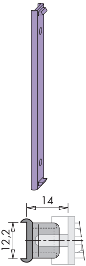
Distanzstück A0002
