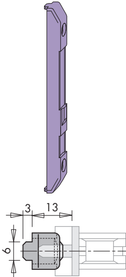
Schließblech A0116
