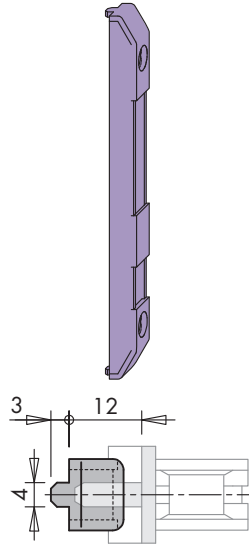
Schließblech A0010
