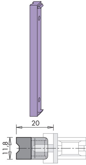
Distanzstück A0008
